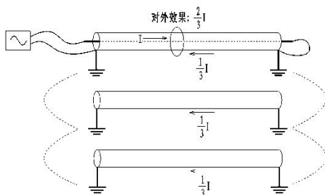
图 5- 10 并行电缆的分流效果
