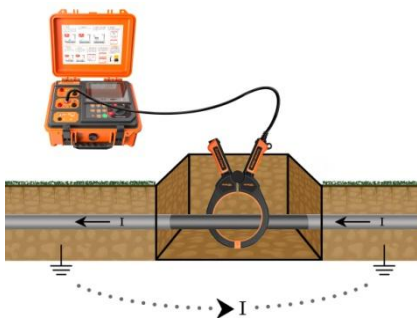
图 5-15 卡钳耦合合法接线图
