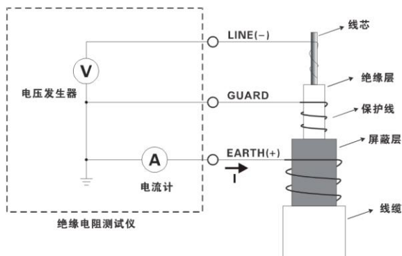
图 8-9 屏蔽端 GUARD 线使用示意图
