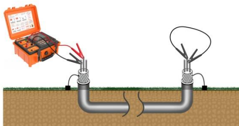
图 5- 11 相间接法接线图
