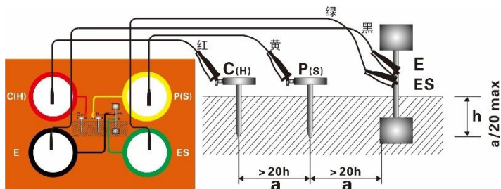
图 8-3 四线法测试接地电阻接线图
