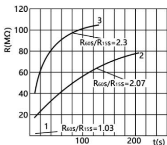
图 8- 10 某台发电机绝缘电阻 R 与实际 t 的关系
