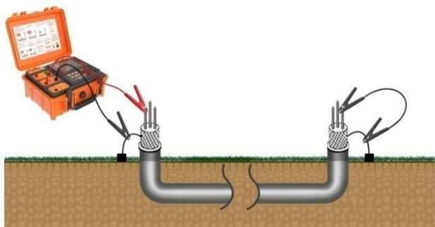
图 5-8 相线-护层接法接线图
