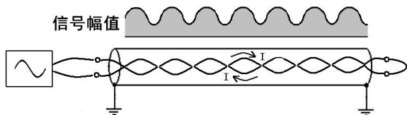
图 5-12 相间接法信号流向示意图
