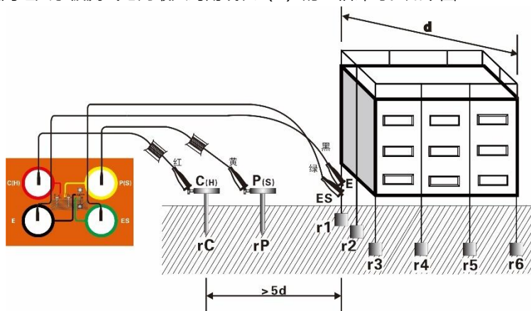
图 8-4 一般楼房地网接地电阻测试接线图
