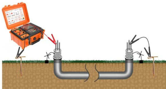
图 5-4 芯线-大地接法接线图
