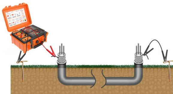
图 5-6 护层-大地接法接线图
