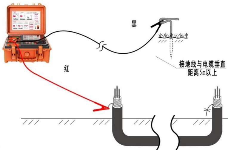
图 8-3 故障定位发射机接线
