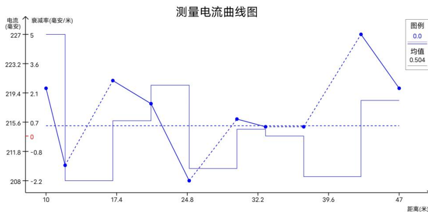
图 7-7 测量电流曲线图
