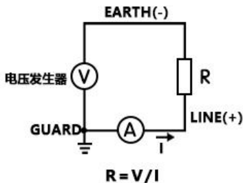
图 8-6 绝缘电阻测量等效电路
