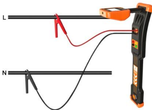
图 8-11 电压测量接线图
