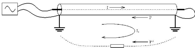
图 5-9 相线-护层接法信号流向示意图
